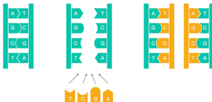
Slika 2.2: Replikacija DNK[12]
