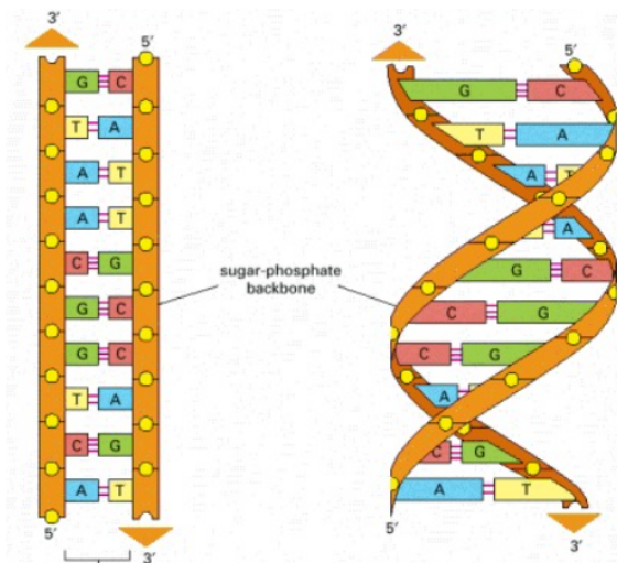
Slika 2.1: Struktura DNK [9]
